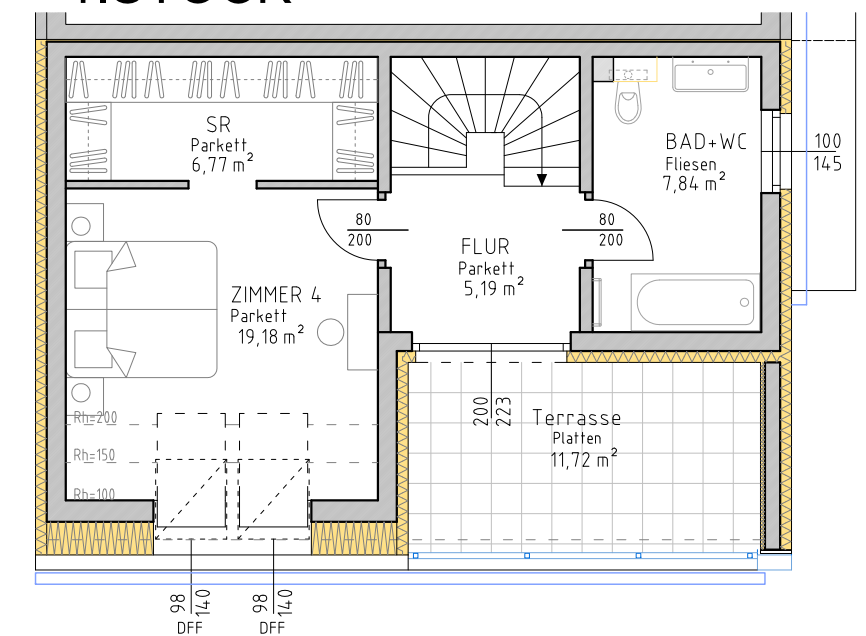
DACHGESCHOSS
